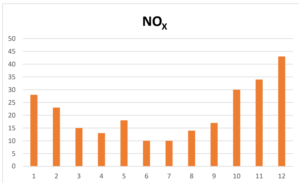
Figura 3: Ossidi di azoto (NO x ): concentrazione media mensile - Stazione di Malagrotta - RM (Anno 2024)
