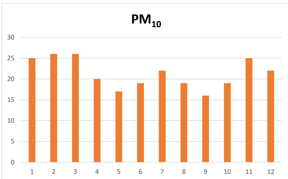
Figura 2: Polveri sottili (PM 10 ): concentrazione media mensile - Stazione di Malagrotta - RM (Anno 2024)
