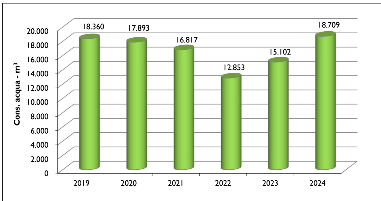
Figura 15: Andamento annuale del consumo di acqua per fini di processo
