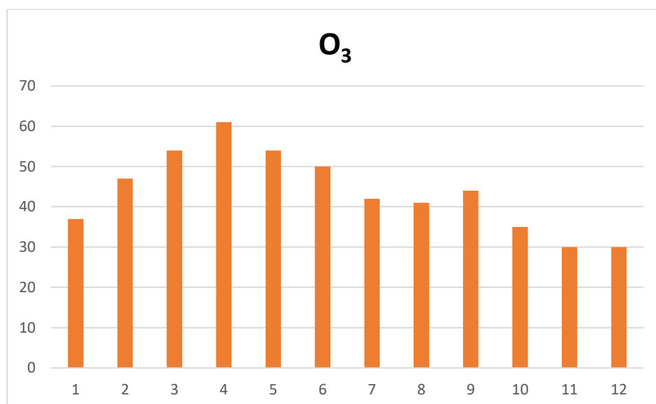
Figura 4: Ozono (O 3 ): concentrazione media mensile - Stazione di Malagrotta - RM (Anno 2024)
