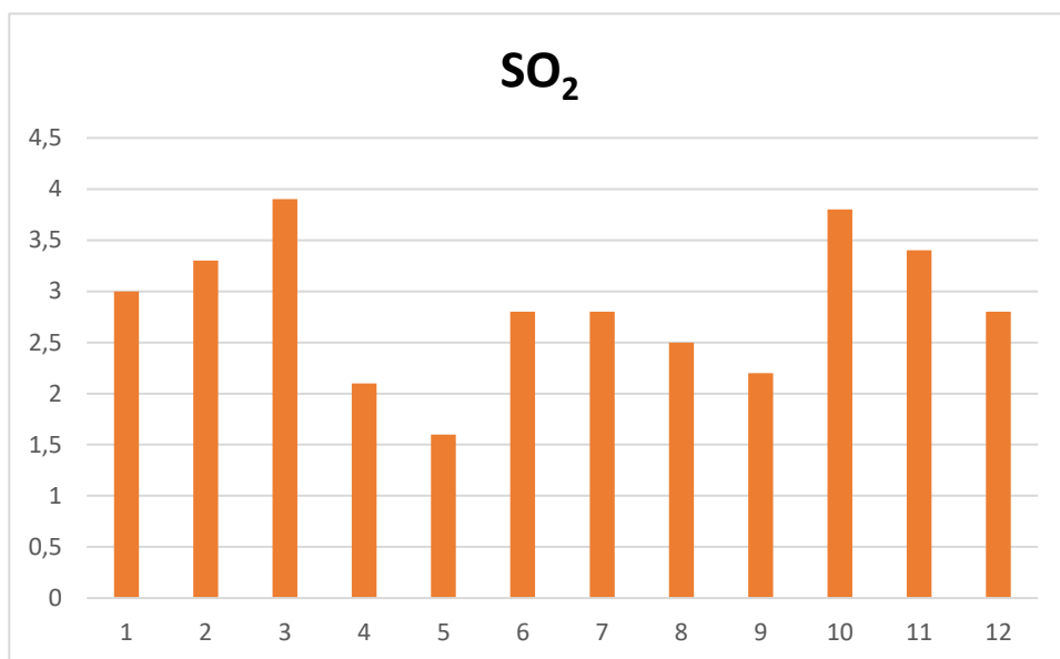
Figura 1: Biossido di zolfo (SO 2 ): concentrazione media mensile - Stazione di Malagrotta - RM (Anno 2024)
