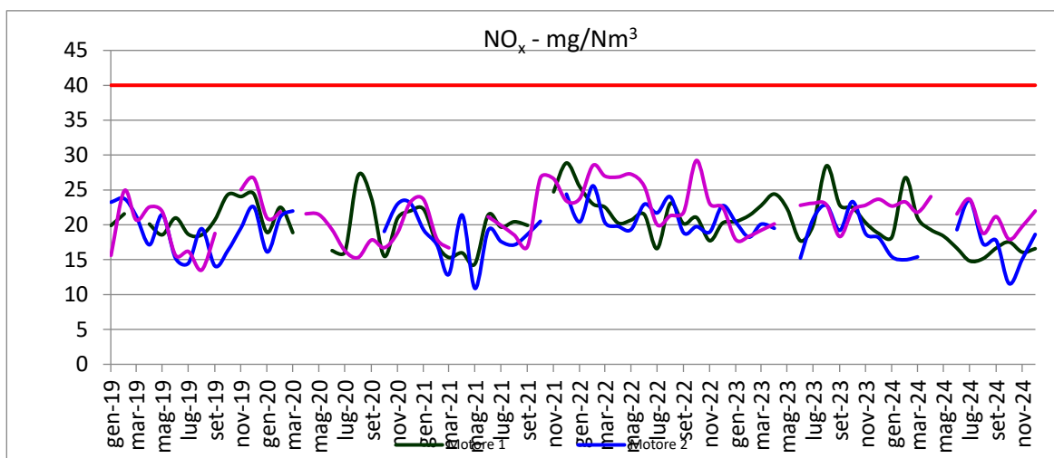
Figura 22: Concentrazioni di Ossidi di Azoto (l'interruzione di una linea indica una media mensile non valida)
